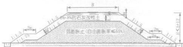
图 1 路基处理图 ( H < 12 + h (m))
