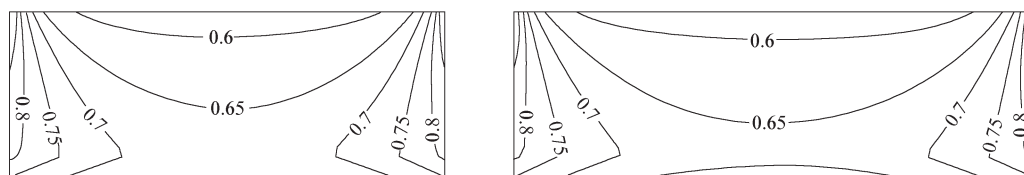
图3 近震时闸基下不同剖面液化指标等值线 ( N_{63.5}=9.7 , \rho_e=5.28\% )
