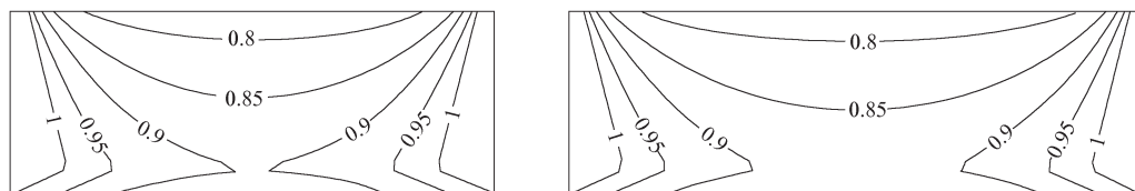
图4 远震时闸基下不同剖面液化指标等值线 ( N_{63.5}=9.7 , \rho_e=5.28\% )
