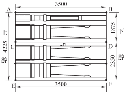
图1 闸室平面
