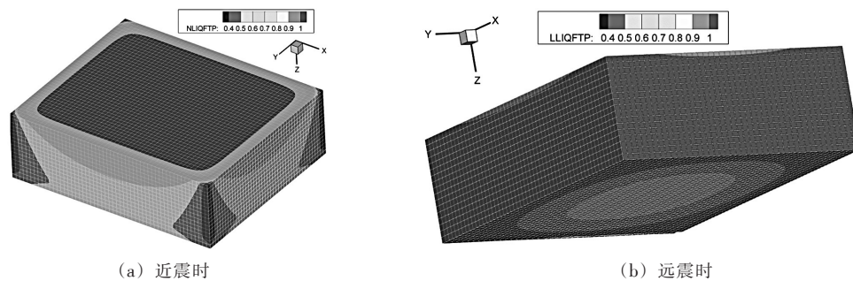
图5 闸基下中细砂层可能液化区域分布云图 ( N_{63.5}=7.6 , \rho_e=5.28\% )
