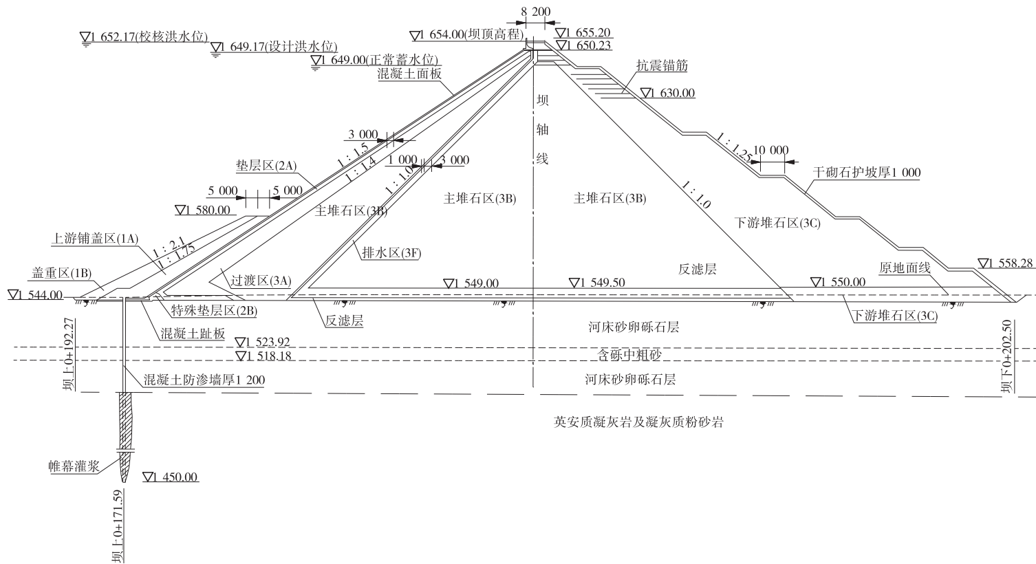
图7 察汗乌苏面板砂砾石坝典型断面图 (单位:高程,m;尺寸,cm)
